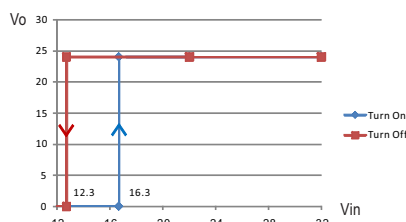
RSD-60L-24
