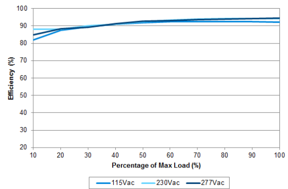
LNE-48V320W□
