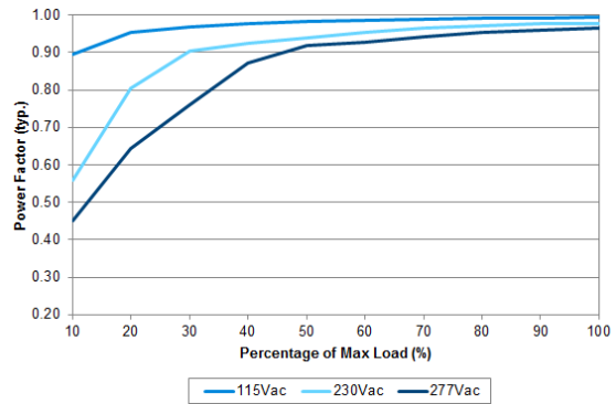
LNE-48V320W□
