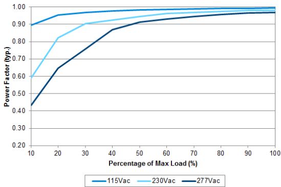
LNE-36V320W□
