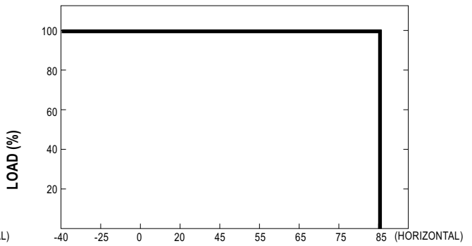
Tcase (°C)
